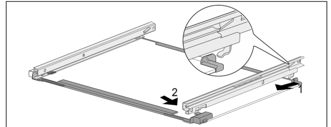
Fig. 158 Скляна пластина з рейками
