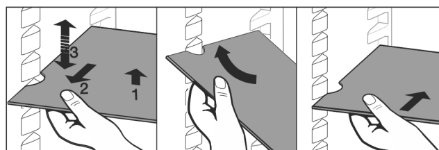
Fig. 123 ► Виймання переставної панелі повністю: витягнути вперед. ► Полегшене виймання: Переставну панель поставити під нахилом. ► Вставка панелей знову: засунути до упору. ► Стопори показують вниз. ► Стопори лежать за передньою знімною полицею. Переставну панель можна також видалити через відділення EasyFresh.
